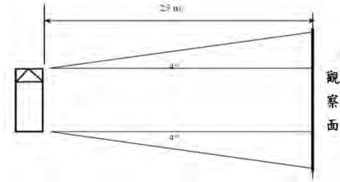
車輛側方反光標識可視性示意圖
