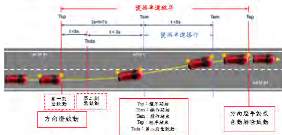
ACSF 類型 C - 側向移動由駕駛以第二刻意致動啟動之案例(二階人機介面)
