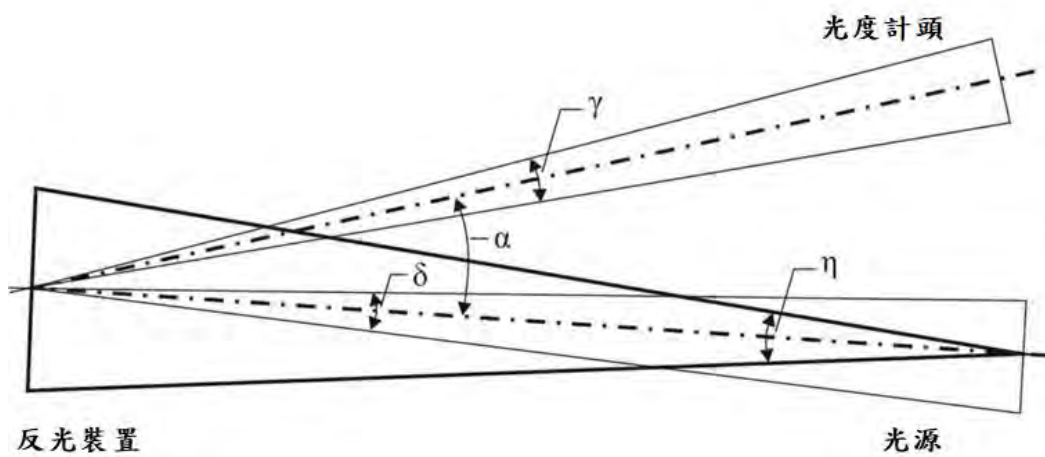
圖三：反光標誌之反光分佈
