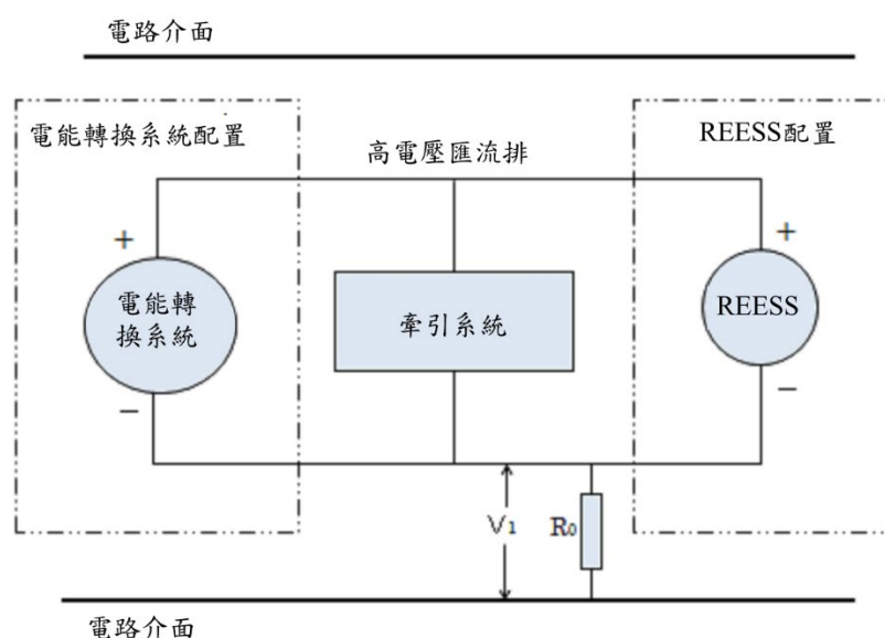
圖 2： V_1' 之量測
