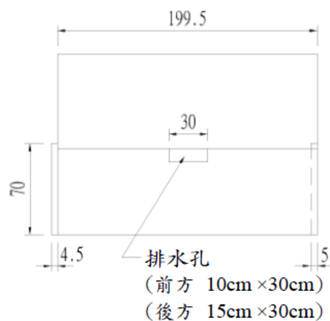
正面示意圖
